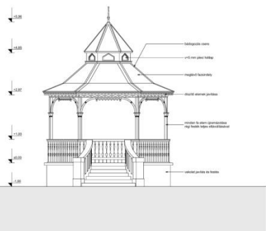
DÉLI NÉZET
