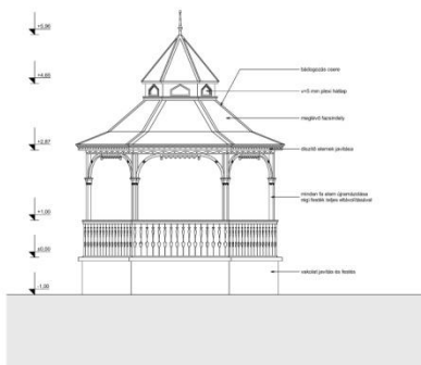
ÉSZAKI NÉZET
